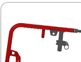
kod 347 rama kompaktowa, kąt ramy przedniej 92°
